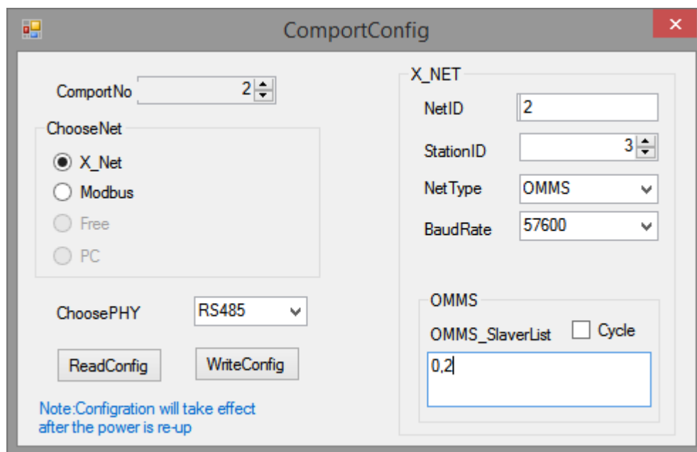
Fig. 3-1 OMMS mode
