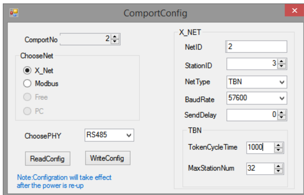
Fig. 3-2 TBN mode
