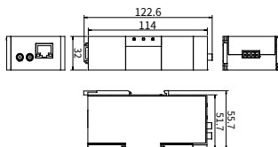
Figura 2-1 Dimensões externas do TBox (Unidade: mm)
