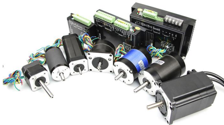
Figura 7 – Motores BLDC e drives de diferentes potências.
