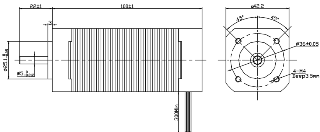
Motor sem escovas KTC-42BLS04-J
