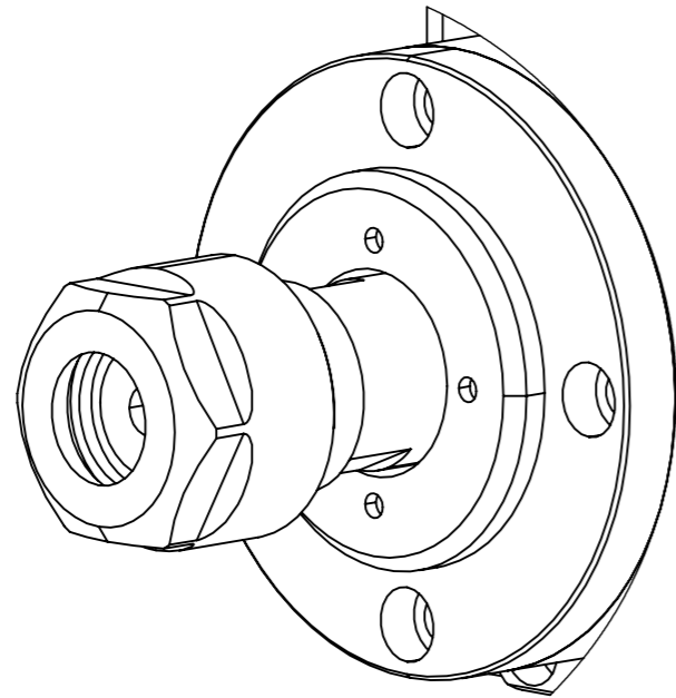
DETALHE B ESCALA 1 : 1
